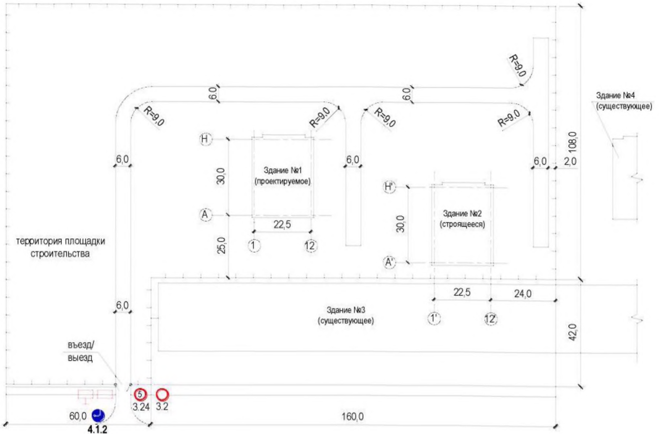
Рис. 6б. Стройгенплан с тупиковыми дорогами
