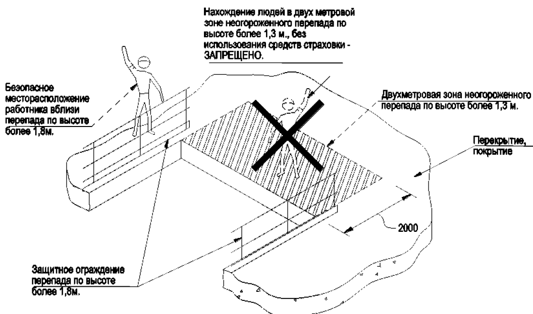
Рис. 38. Схемы по безопасному ведению работ в двухметровой зоне неогороженного перепада по высоте более 1,8м.
