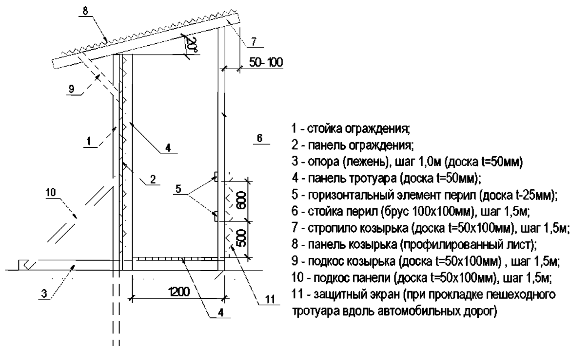
Рис. 2. Схема устройства защитного козырька
